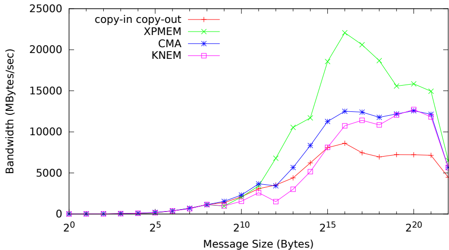
IMB Sendrecv Bandwidth (IMB Sendrecv)
